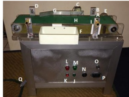
Gambar 5. Konveyor input tampak depan
