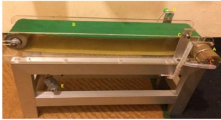
Gambar 7. Konveyor pengepakan
