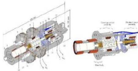
Gambar 1. Mesin stirling tipe free piston
