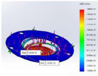
Gambar 10. Displacement
