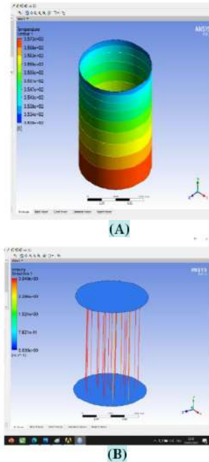
Gambar 5. Hasil simulasi (A) gambar distribusi pada regenerator; (B) kecepatan aliran fluida pada regenerator
