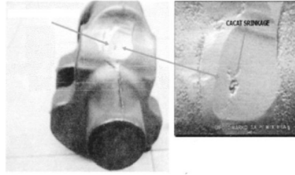
Gambar 6. Poros engkol yang mengalami cacat macro shrinkage
