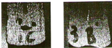
Gambar 2. Identifikasi cacat macro shrinkage pada riser
