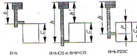
Gambar 4. Penentuan tinggi efektif logam cair
