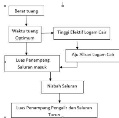
Gambar 3. Diagram alir perhitungan perancangan pengecoran
