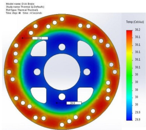
Gambar 2. Hasil simulasi termal
