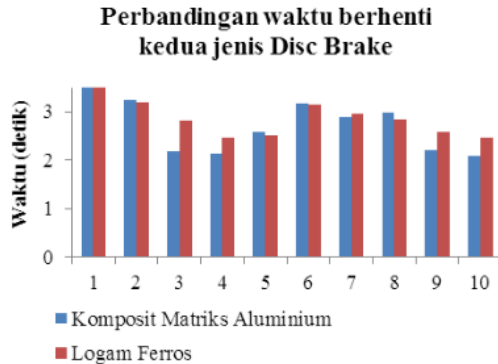
Gambar 4.14. Perbandingan waktu berhenti kedua jenis disc brake
