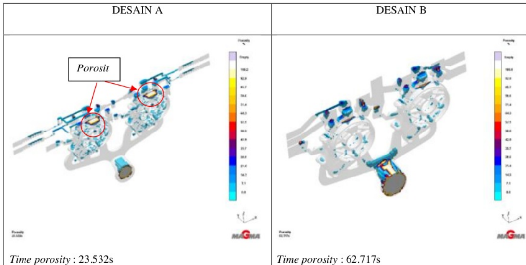
Gambar 9. hasil proses simulasi magma
