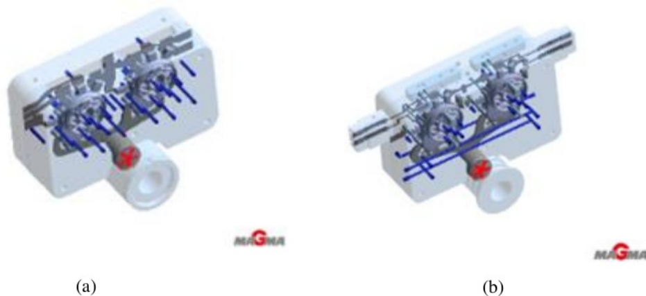
Gambar. 3. Desain geometry (a) desain geometry pada posisi awal, (b) desain geometry perubahan pada gate dan pembesaran pada biskuit gambar geometri sebelum di lakukan simulasi pada software magma V
