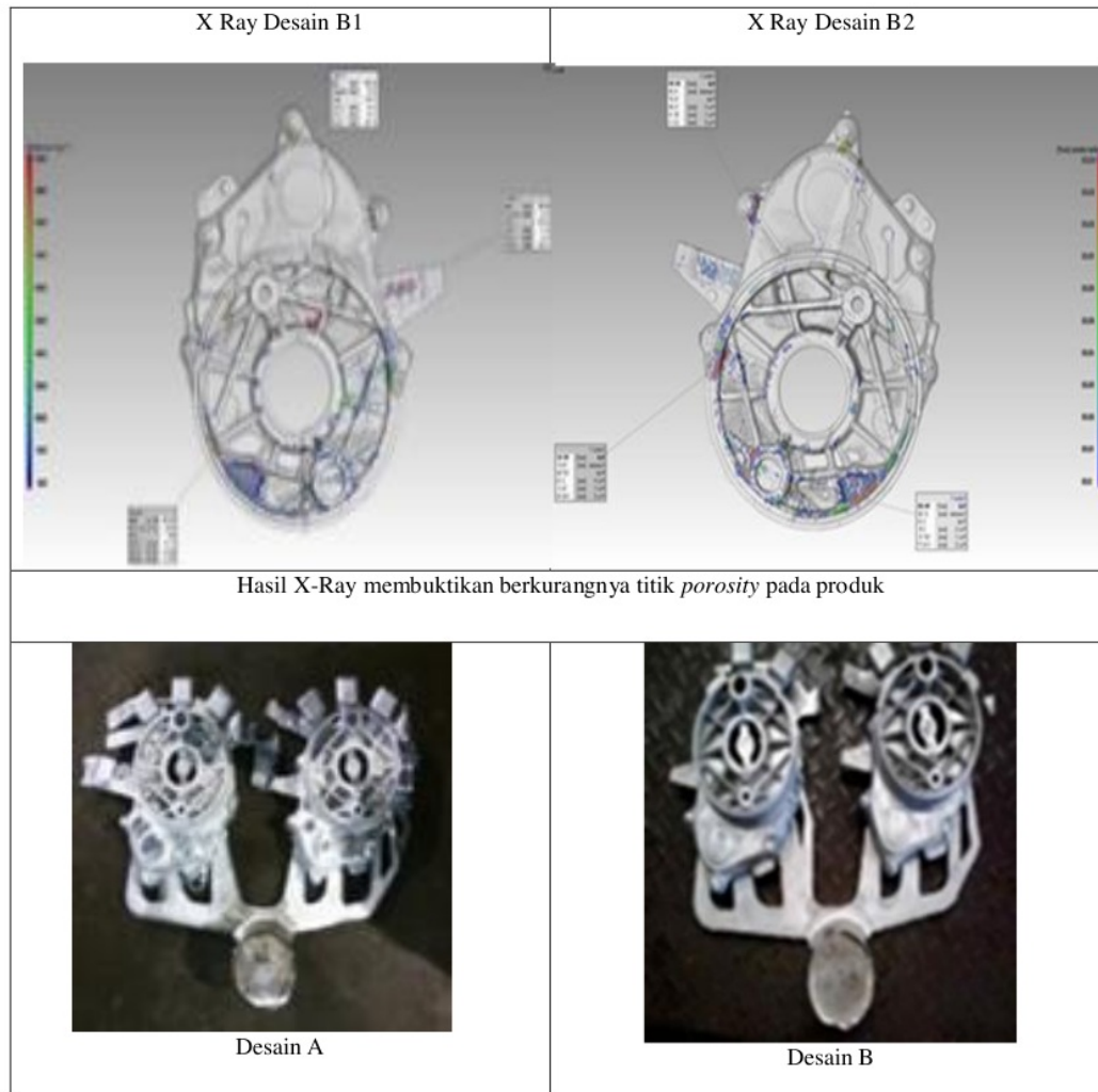
Gambar 10. hasil analisa dengan X-Ray
