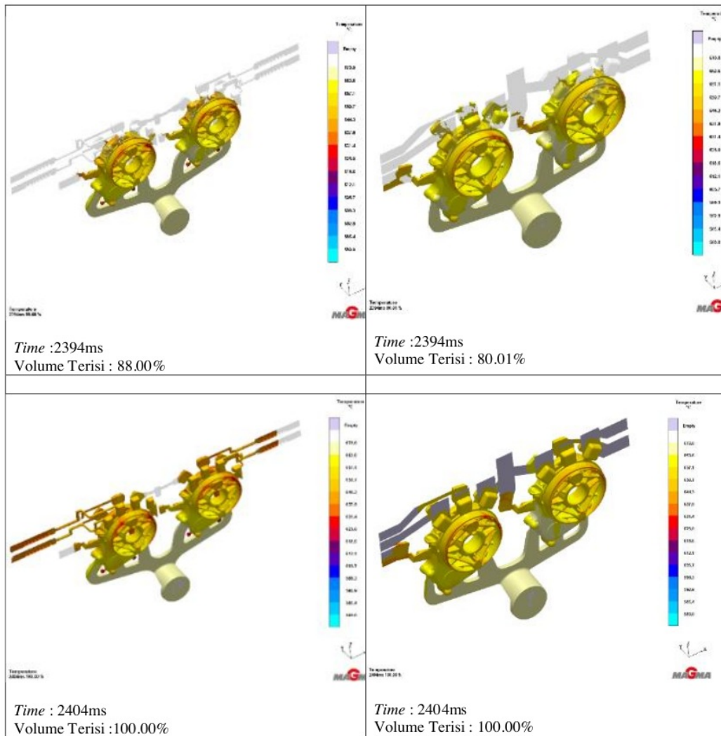
Gambar 4. Hasil Simulasi Pengisian Dies
