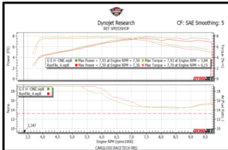
Gambar 6. Hasil Uji Power, Torque, dan AFR
