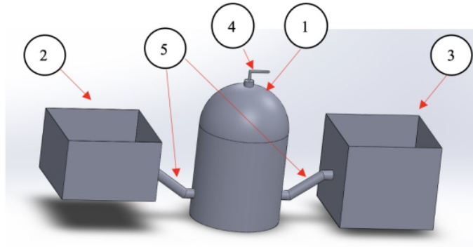
Gambar 12. Komponen-komponen biodigester fixed dome
