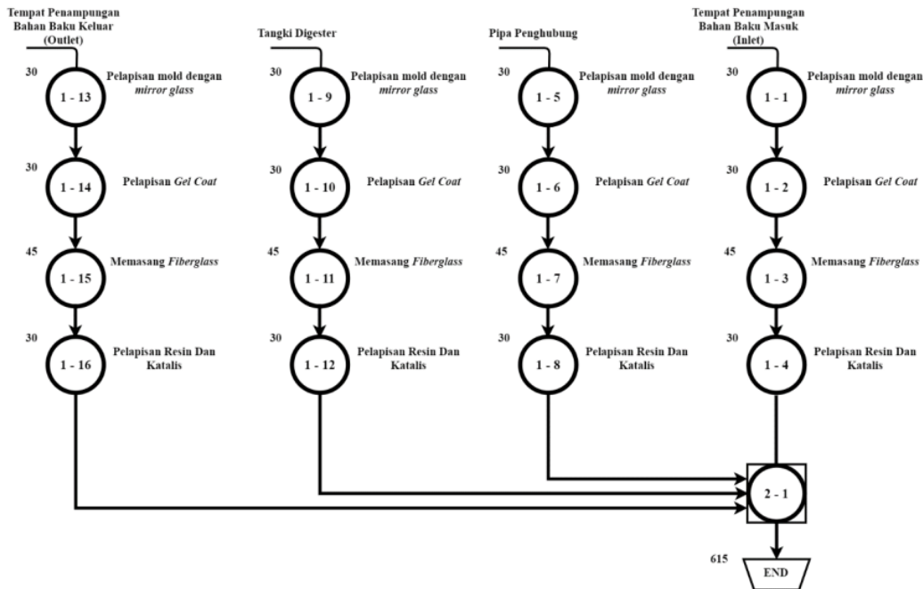
Gambar 17. OPC biodigester tipe fixed dome
