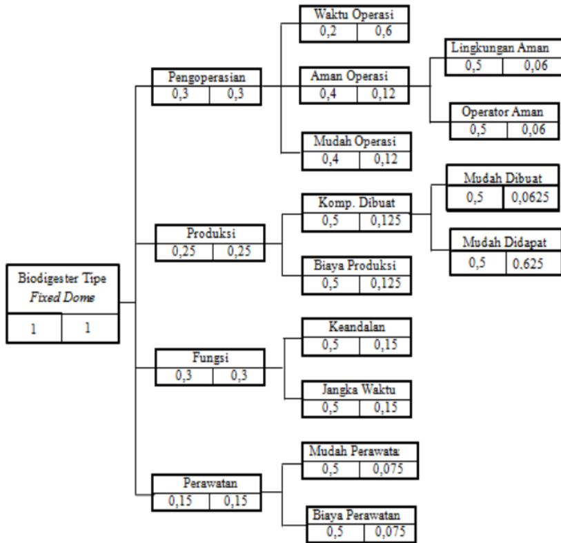
Gambar 10. Pohon keputusan
