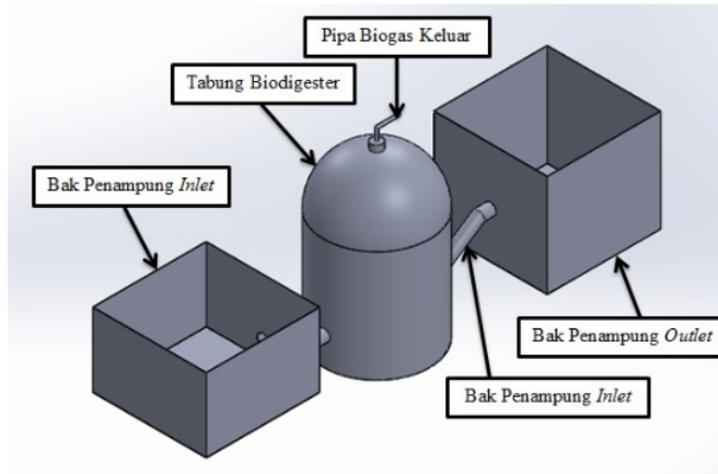
Gambar 11. Desain biodigester tipe fixed dome
