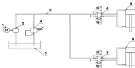
Gambar 2 Sirkuit Hidrolik
