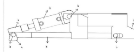
Gambar 6. sistem pengangkat hidrolik tampak samping
