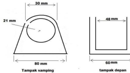
Gambar 15. Kaki Penyangga
