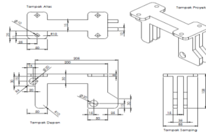
Gambar 12. Rangka Utama Pegangan Silinder dan Lengan
