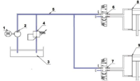
Gambar 3 Posisi Netral Pada Sirkuit Hidrolik
