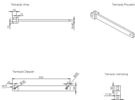
Gambar 14. Lengan
