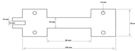
Gambar 13. Plat Penyangga Atas
