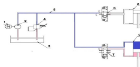
Gambar 4 Posisi ketika katup kontrol terbuka
