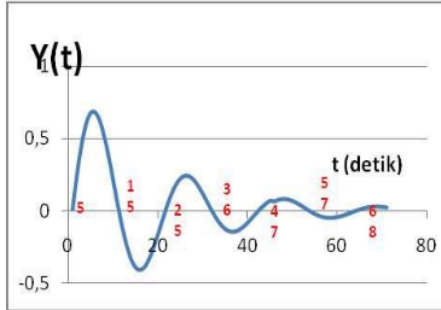
Gambar 3 Persamaan Getaran Paksa Dengan Peredam Eksperimen 1, 9, 10 dan 13
