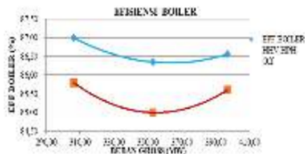
Gambar 6. Grafik Efisiensi Boiler Terhadap Beban Gross
