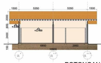
POTONGAN 1
