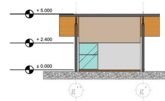
TAMPAK BELAKANG KANTOR
