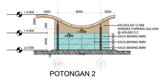
POTONGAN 2
