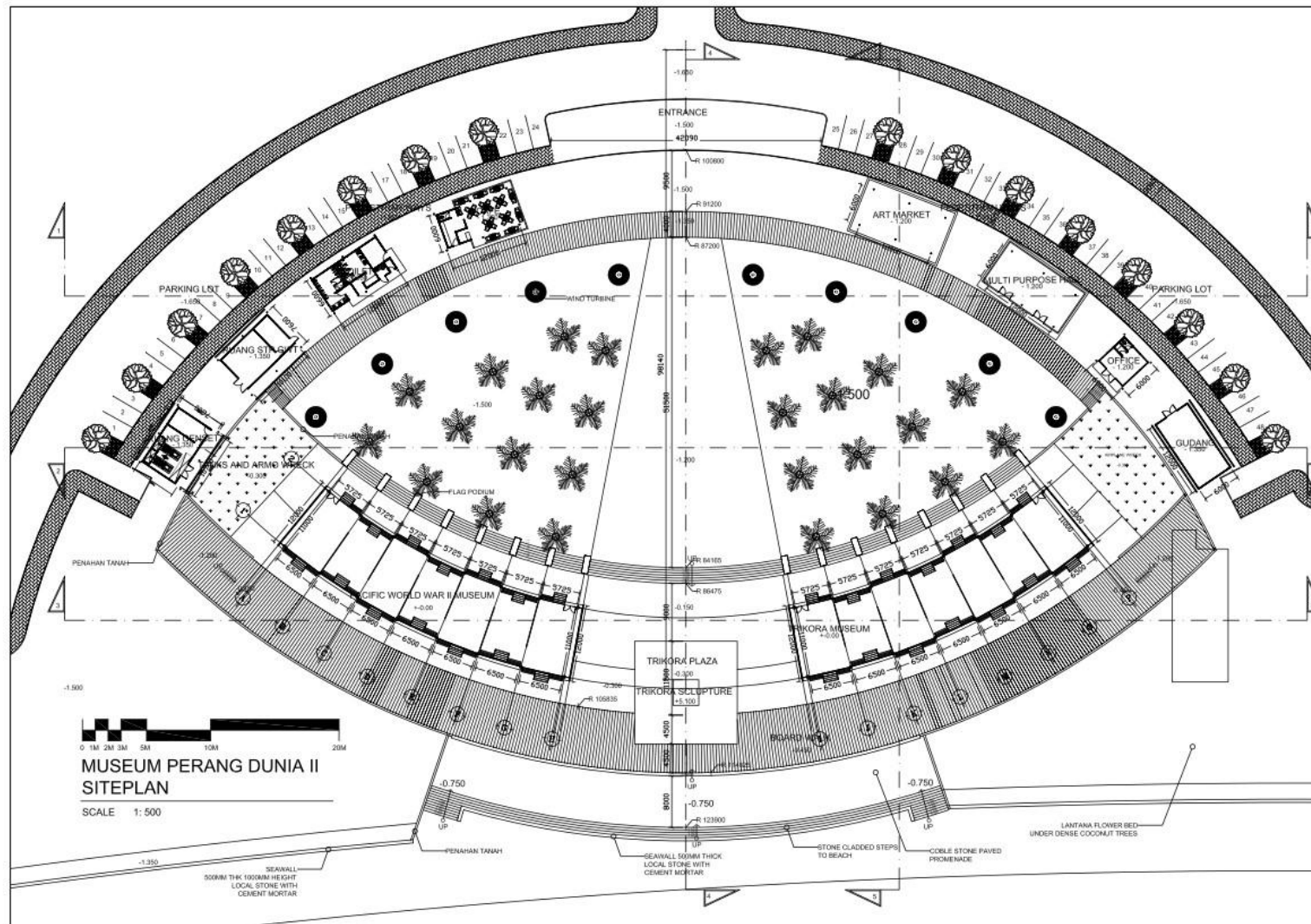
SITEPLAN
