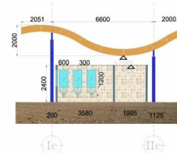
POTONGAN 2
