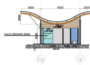
POTONGAN 1
