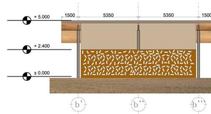
TAMPAK DEPAN RUANG STP GWT
