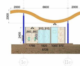
POTONGAN 1
