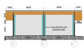
POTONGAN 1
