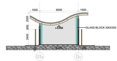
POTONGAN 2
