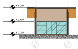
TAMPAK DEPAN KANTOR
