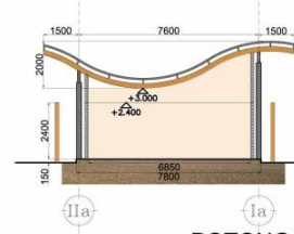
POTONGAN 2
