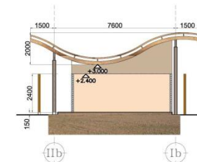
POTONGAN 2
