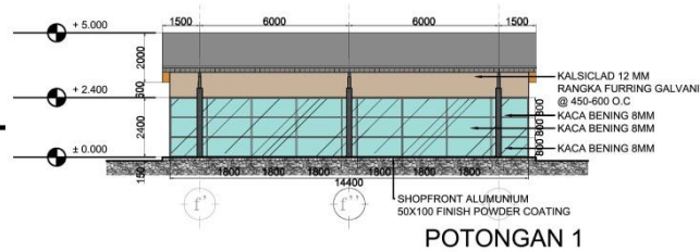
POTONGAN 1
