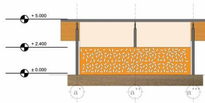
TAMPAK DEPAN RUANG GENSET
