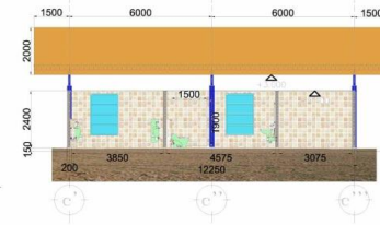
POTONGAN 3
