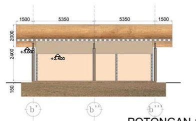
POTONGAN 1
