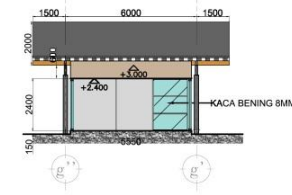
POTONGAN 2
