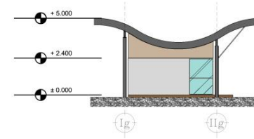
TAMPAK KIRI KANTOR
